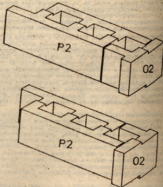
Łączenie pustaków w systemie „Centrum” budownictwa indywidualnego.
