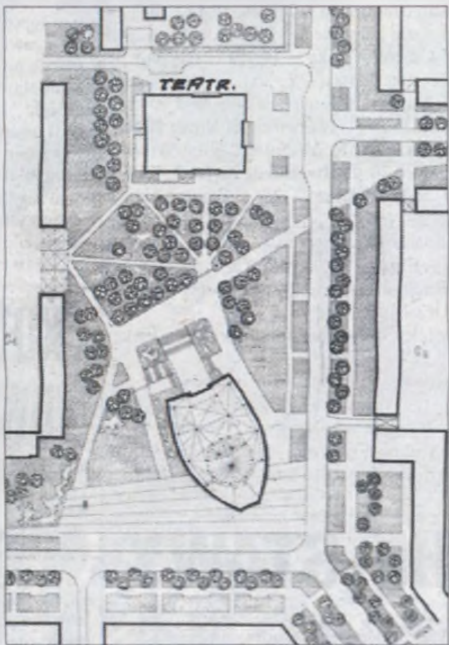
Plan lokalizacji kościoła na osiedlu C-1 (Teatralne), I Nagroda w konkursie SARP w 1957 r. Fot. autor nieznany, Miastoprojekt – Kraków, ze zbiorów Arkadiusza Sitarskiego.
