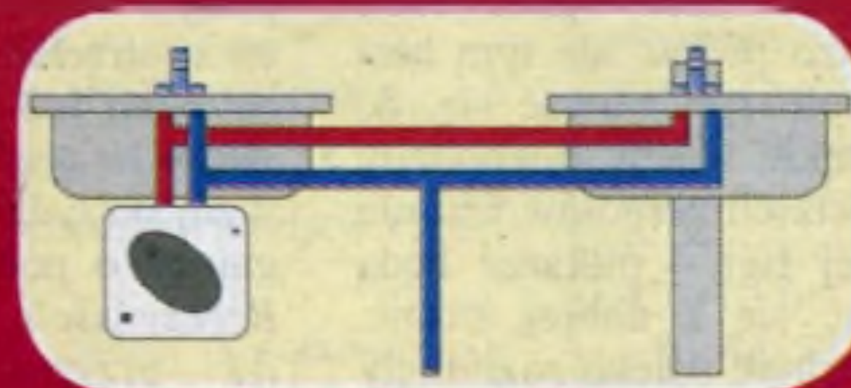
Rys. 1 – SYSTEM NIEZALEŻNY podgrzewacz jako jedyne źródło ciepłej wody
