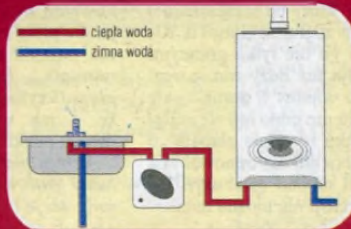
Rys. 2 – SYSTEM SZEREGOWY podgrzewacz podłączony za innym źródłem ciepłej wody
