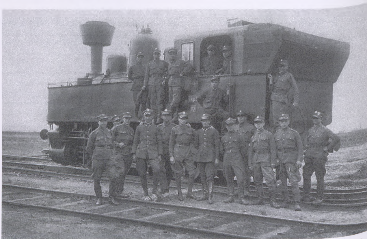
Austriacki parowóz serii TKp11-12, pracujący przed wojną na kolei kocmyrzowskiej w barwach PKP. Fotografia z maja 1930 r. z linii Kraków-Kocmyrzów. Fot. ze zbiorów Piotra Skuchy
