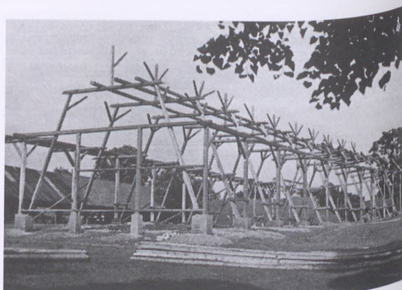
Konstrukcja stodoły odbudowywanej po pożarze przez ekipę Jakuba Bębna w majątku cysterskim, 1938 r.
