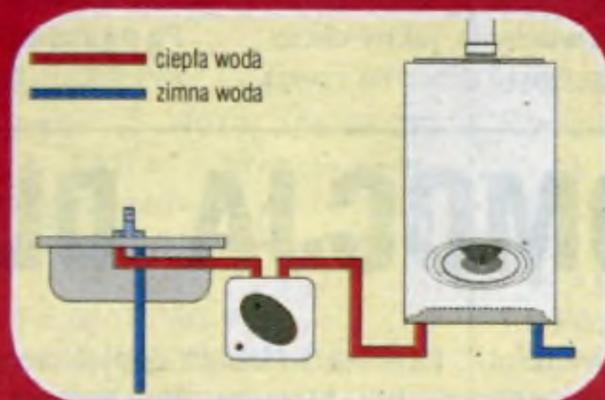
Rys. 2 – SYSTEM SZEREGOWY podgrzewacz podłączony za innym źródłem ciepłej wody
