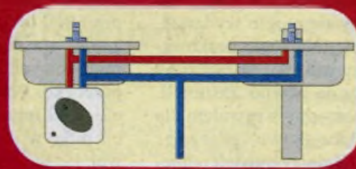
Rys. 1 – SYSTEM NIEZALEŻNY podgrzewacz jako jedyne źródło ciepłej wody
